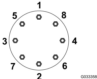
Bild 10 Vorderräder
