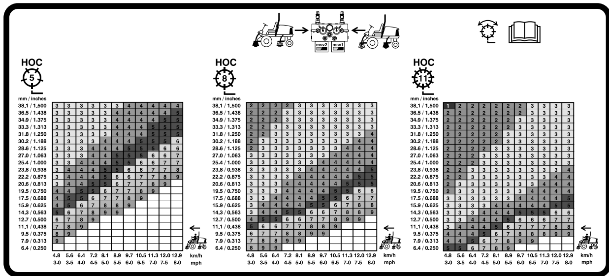
図 42 5 インチ 127mm リールの速度表
