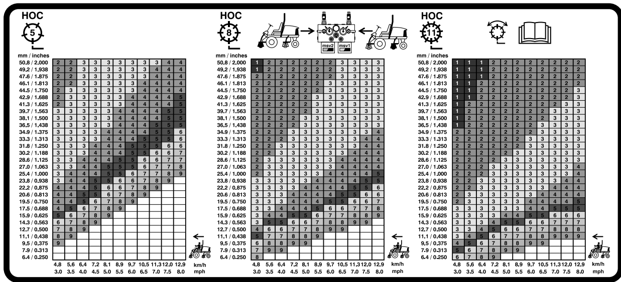
図 43 7 インチ177.8mmリールの速度表
