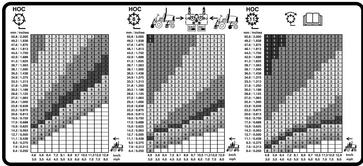
Figuur 34 Tabel met toerentallen voor messenkooien van 178 mm
