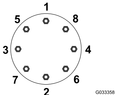
Bild 12 Vorderräder
