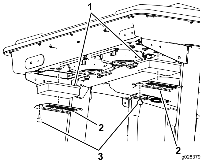
Bild 90 Hinterer Kabinenluftfilter
