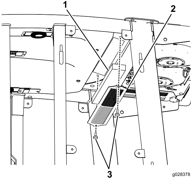
Bild 89 Interner Kabinenluftfilter
