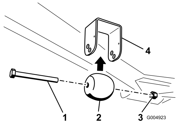
Kuva 26 Vain Guardian-leikkuupöydät
