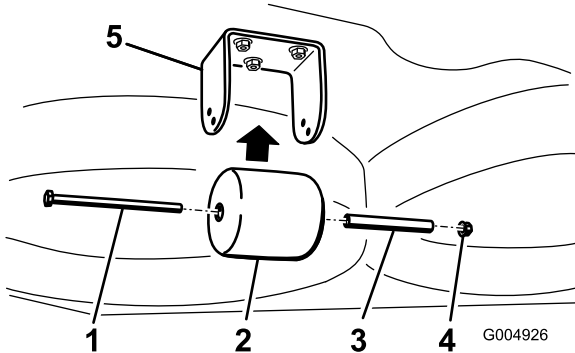
Kuva 25 Vain Guardian-leikkuupöydät
