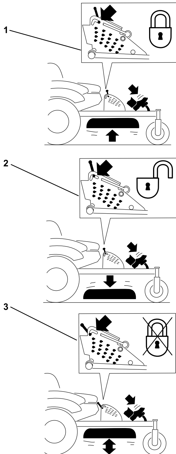
Figur 26 Transportlåsstillinger
