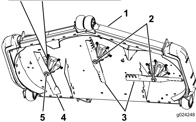
Kuva 97 Terän sijainti
