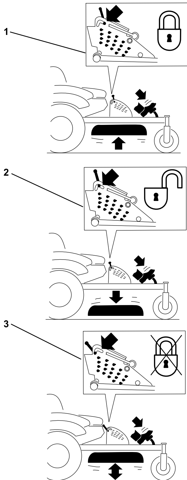
Kuva 26 Kuljetuslukon asennot
