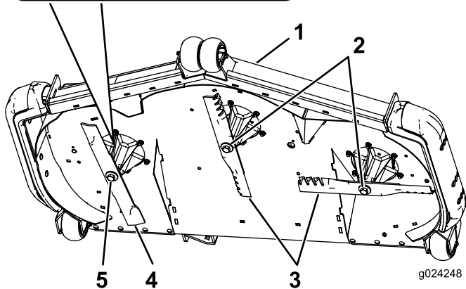
Kuva 93 Terän sijainti
