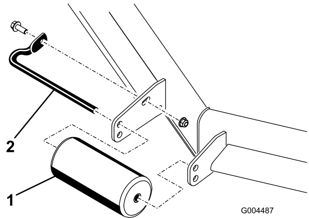
Figur 24 Alla klippdäck
