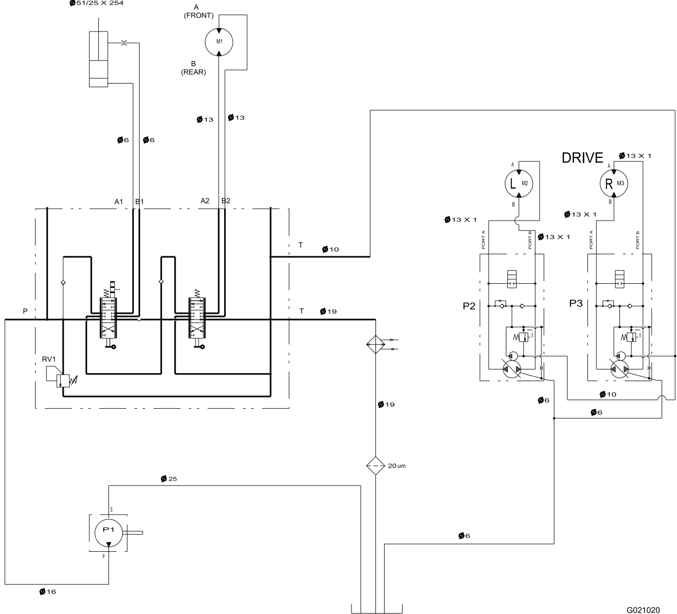
Schema idraulico (Rev. B)
