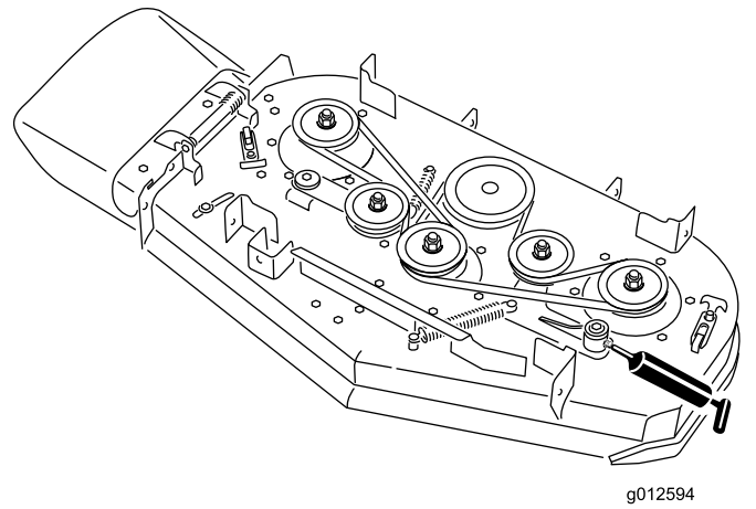
Kuva 37 102 cm:n leikkuupöytä
