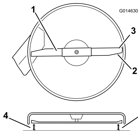
Figuur 50 Maaidekken met één mes
