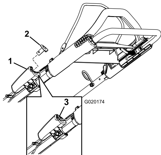
Figura 13 Arrancador eléctrico
