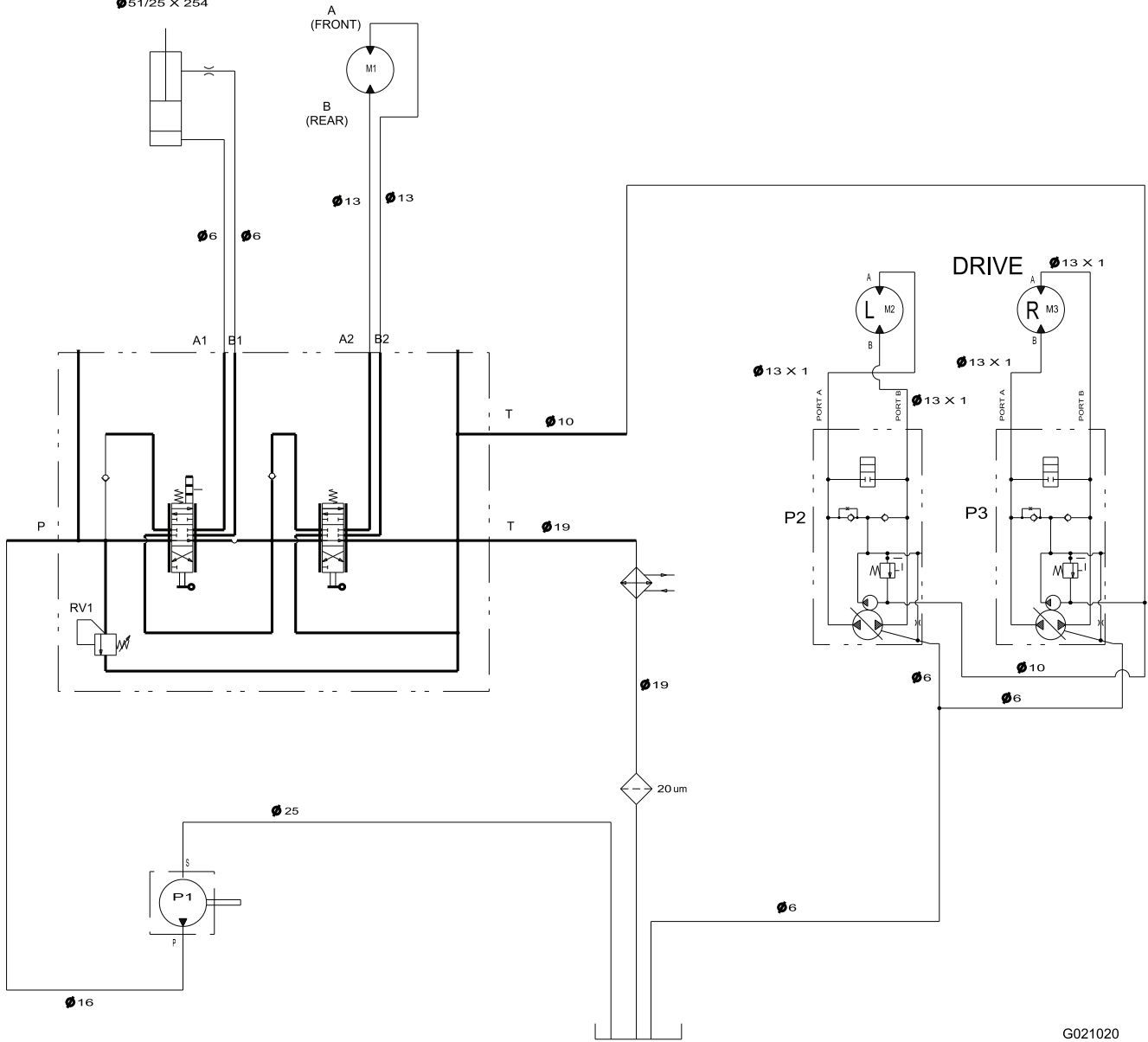
Hydraulikschemata (Rev. B)
