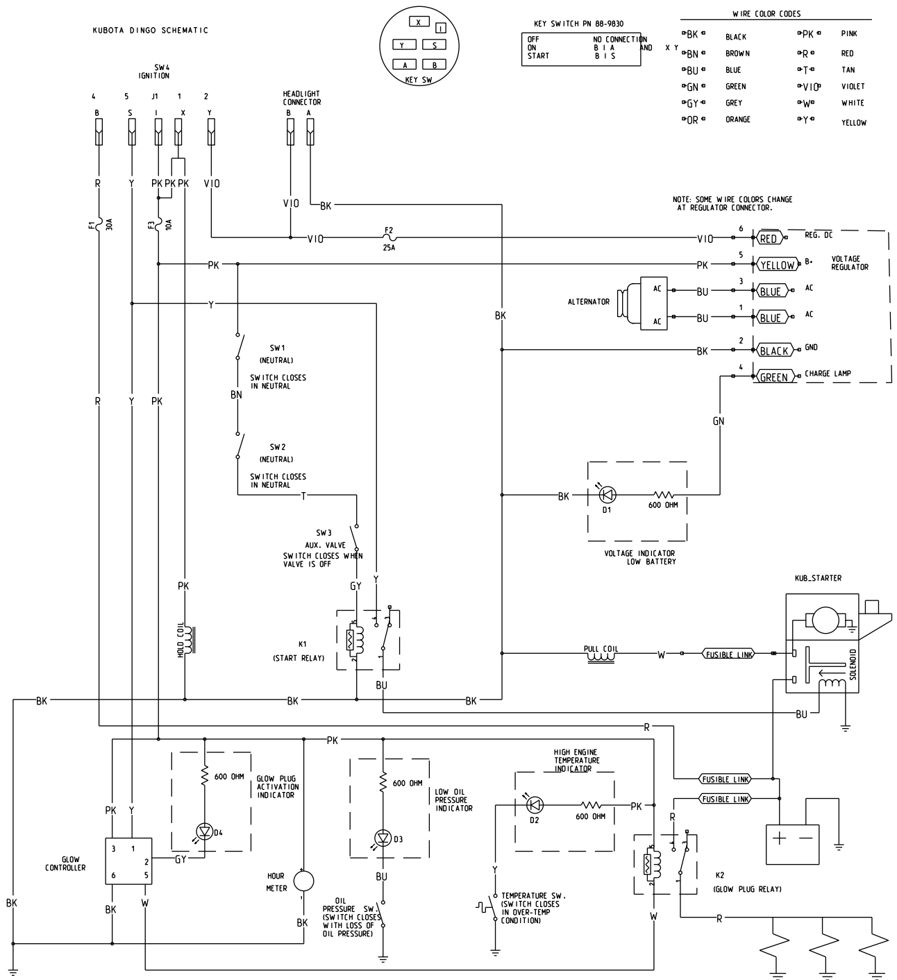
Elektrické schéma (Rev. A)
