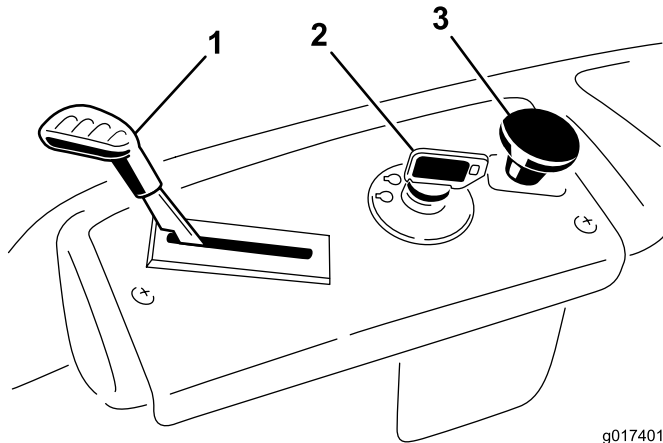
Kuva 5 Ohjauspaneeli
