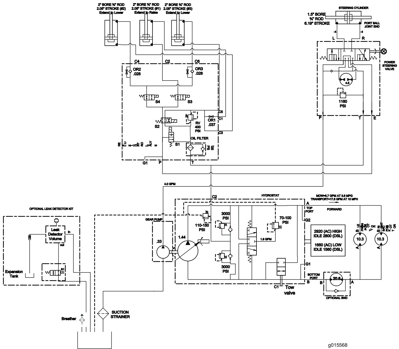
Hydraulisches Schema (Rev. A)
