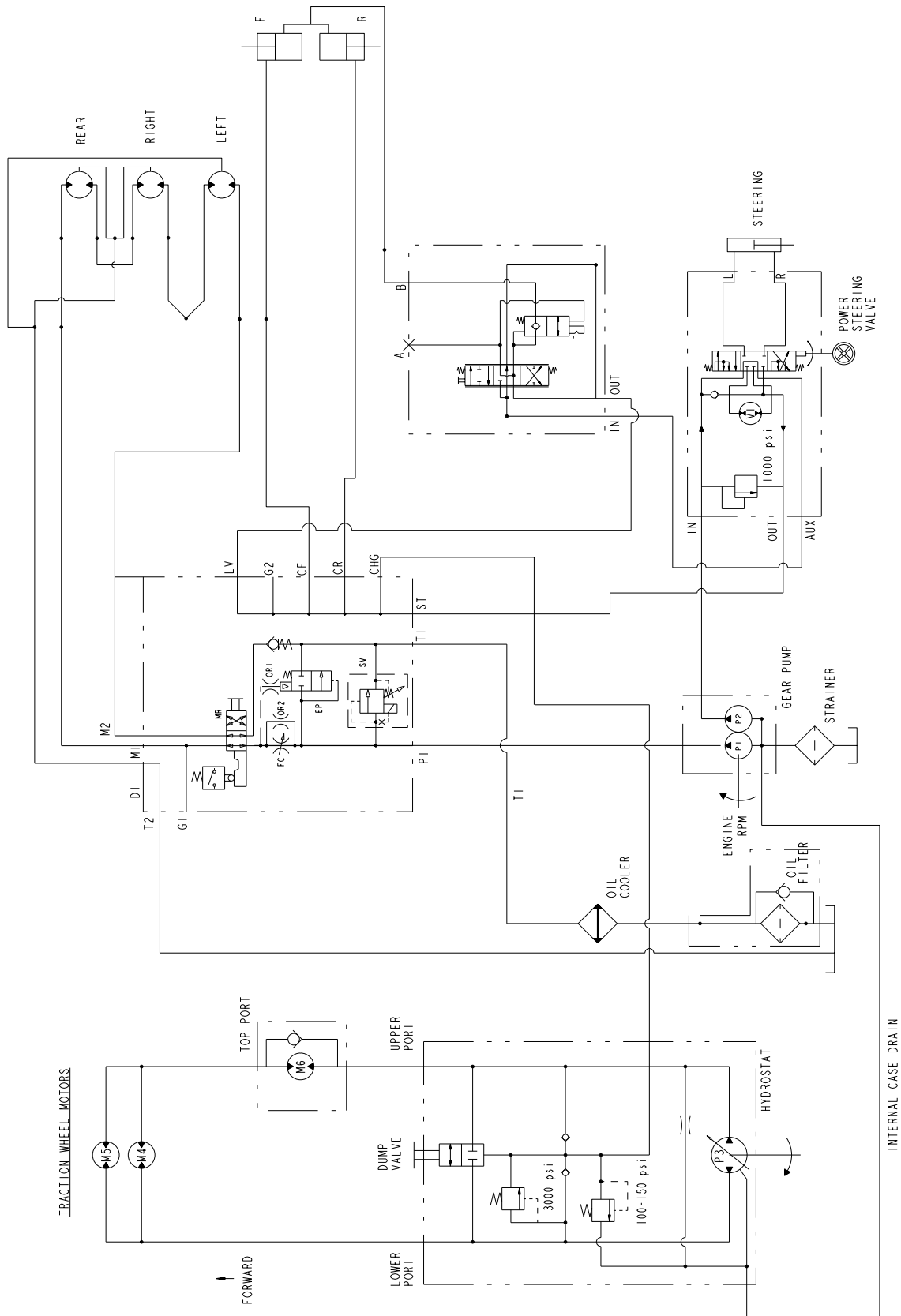
Esquema hidráulico-Modelo 03170 (Rev. A)
