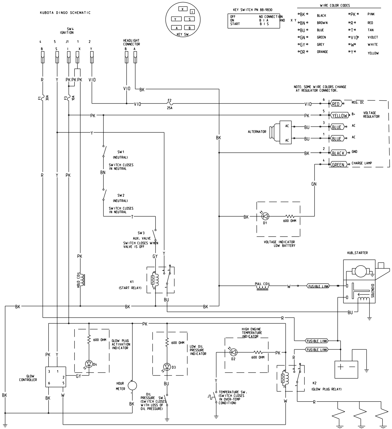
Schema elettrico (Rev. A)
