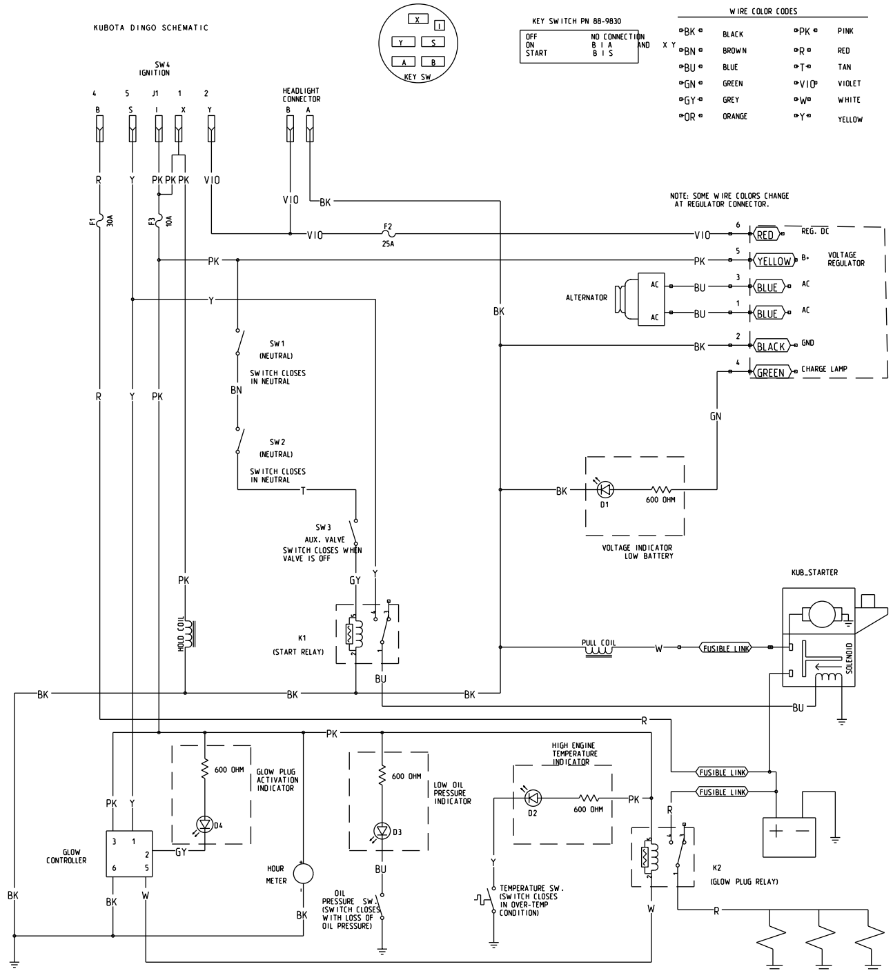
Esquema eléctrico (Rev. A)
