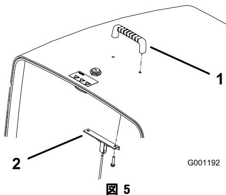
1. ハンドル 2. フードケーブルブラケット
