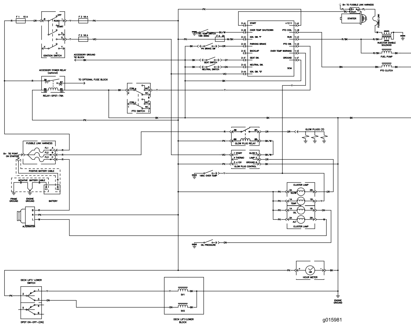
電気回路図 (Rev. A)
