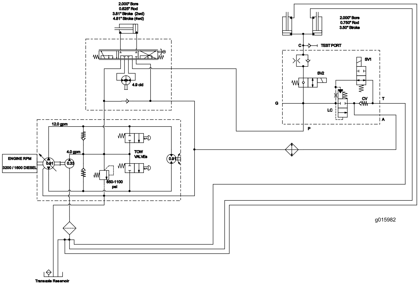
油圧回路図 (Rev. A)
