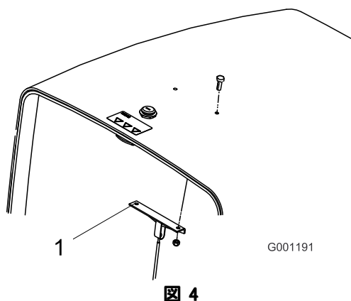
1. フードケーブルブラケット
