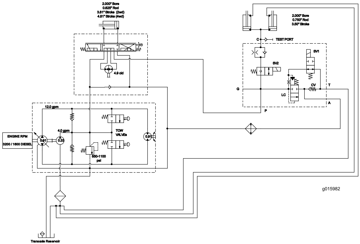
Schema idraulico (Rev. A)
