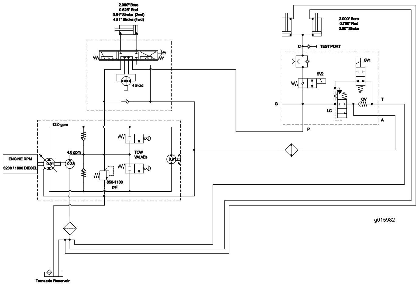
Schéma hydraulique (Rev. A)
