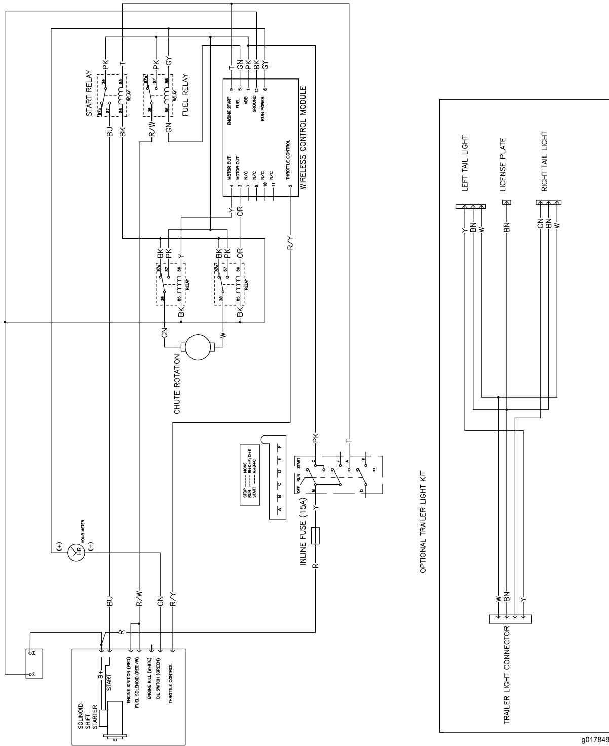
Ledningsdiagram (Rev. -)
