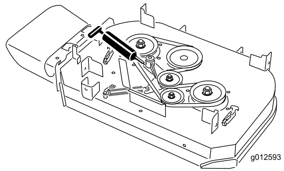
Bild 37 91-cm-Mähwerk
