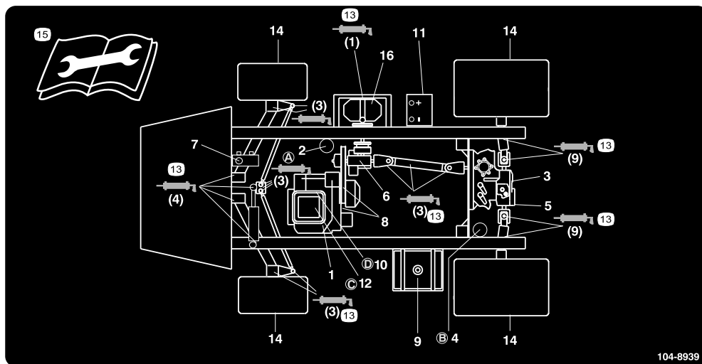
Bild 32 Wartungsstellen
