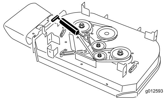
Figura 36 Carcasa de corte de 36 pulgadas (91 cm)
