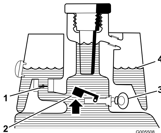
Figur 29 Normal drift (varm olja)
