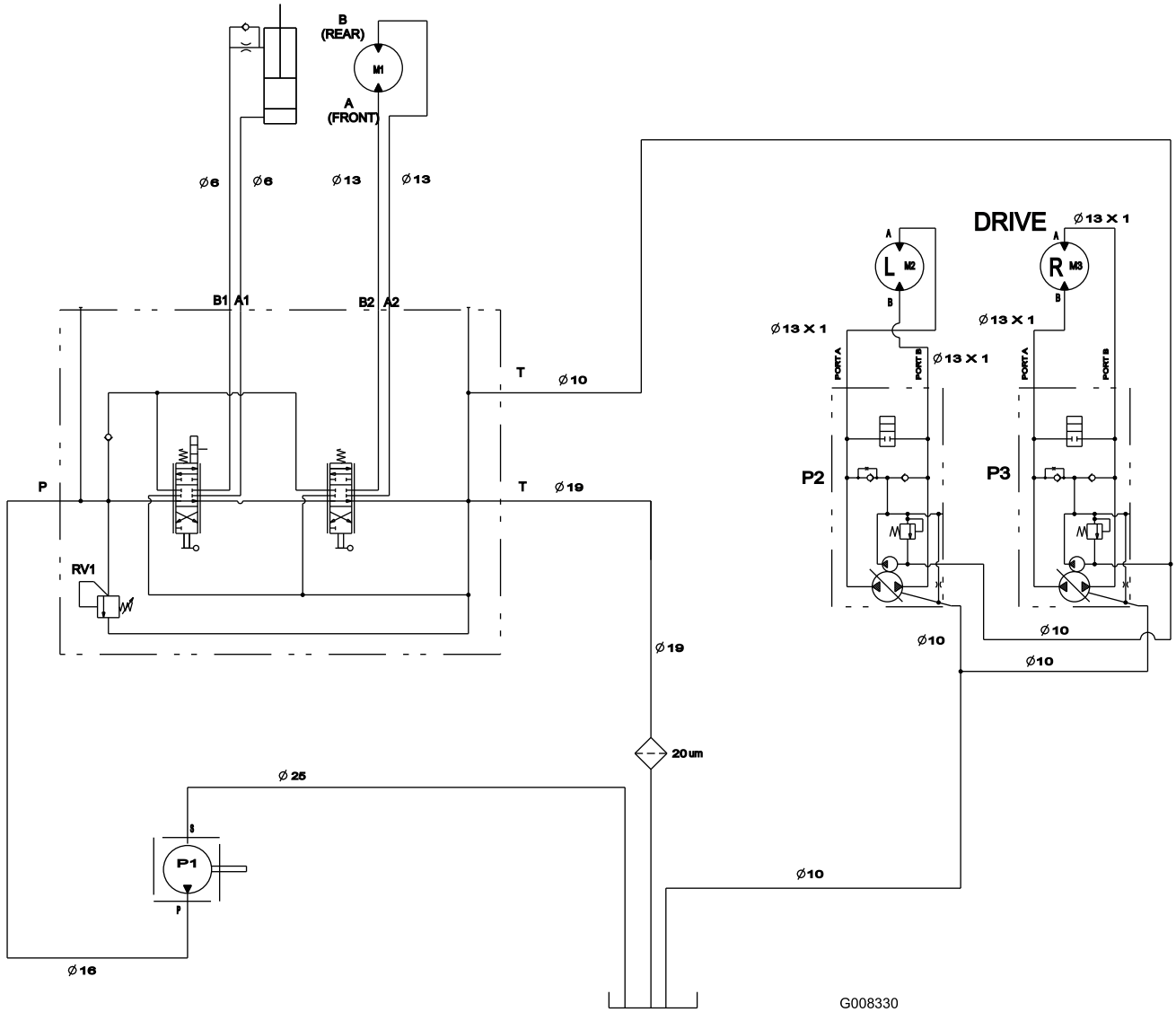
Schema Idraulico - Modello 22970 (Rev. A)
