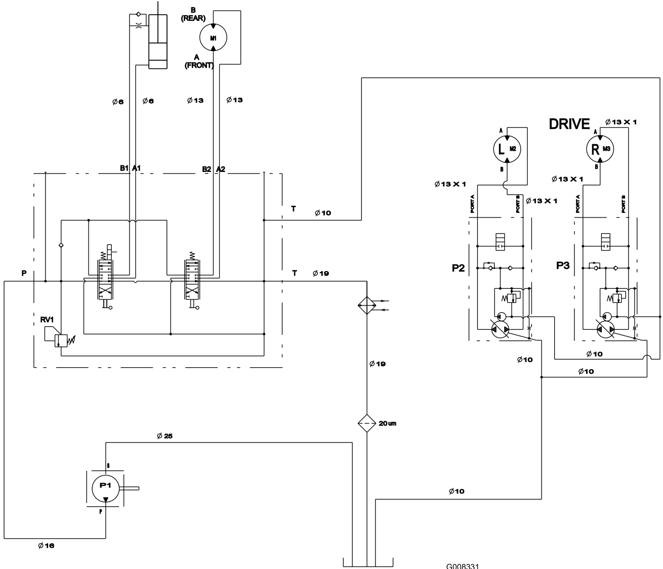
Esquema hidráulico—Modelo 22971 y 22974 (Rev. A)
