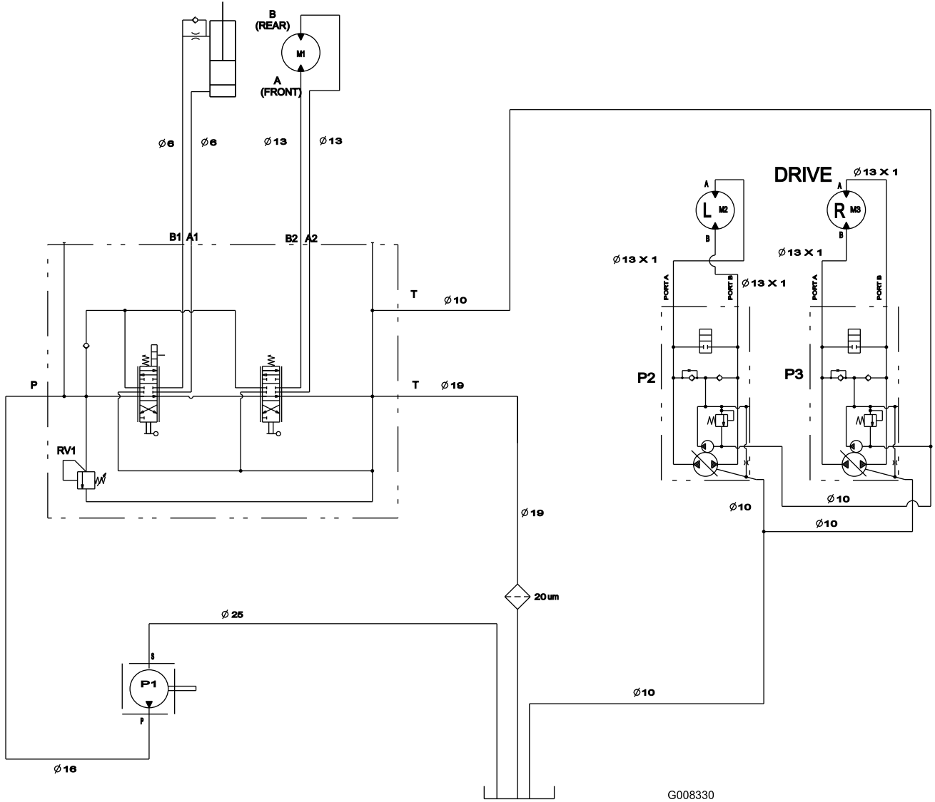
Esquema hidráulico—Modelo 22970 (Rev. A)
