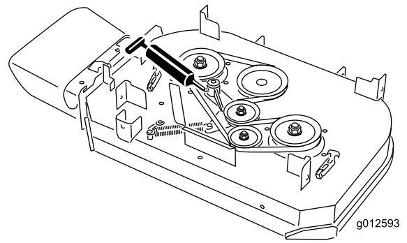
Figura 36 Plataforma de corte de 36 pulgadas (91 cm)
