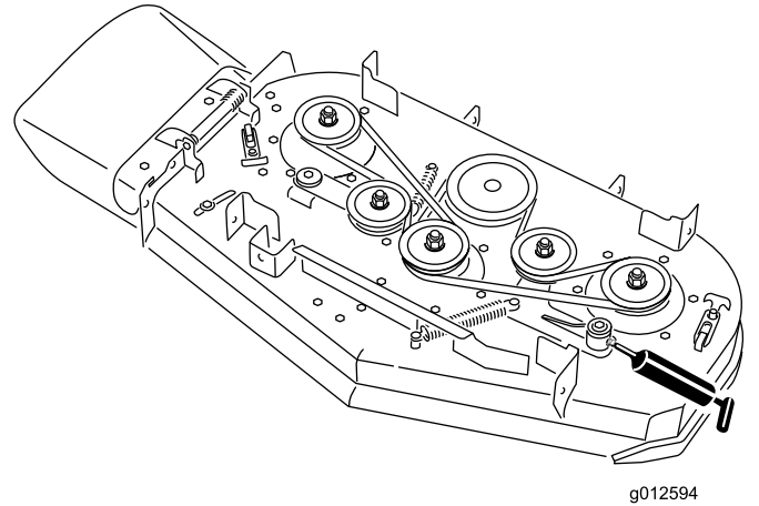
Figura 37 Plataforma de corte de 40 pulgadas (102 cm)
