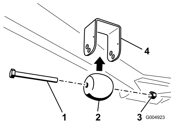
Figuur 30 Uitsluitend Guardian-maaidekken
