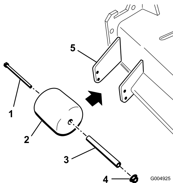
Figuur 31 Uitsluitend maaidekken met zijafvoer
