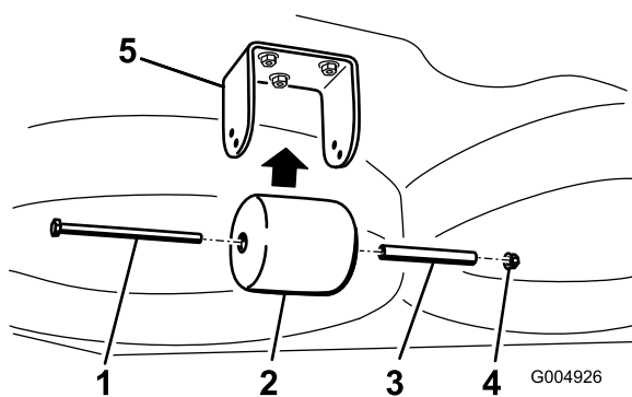
Kuva 29 Vain Guardian-leikkuupöydät
