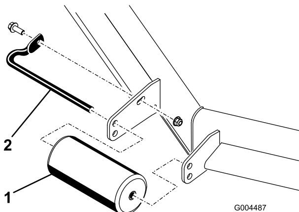
Kuva 28 Kaikki leikkuupöydät
