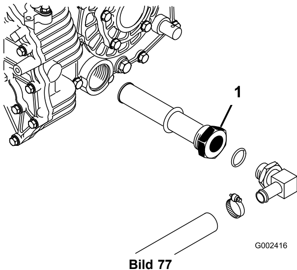
1. Hydrauliksieb
