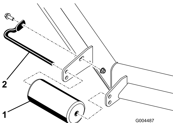
Figur 27 Alle klippeenheter
