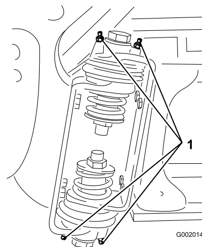
Figur 43 Højre bom
