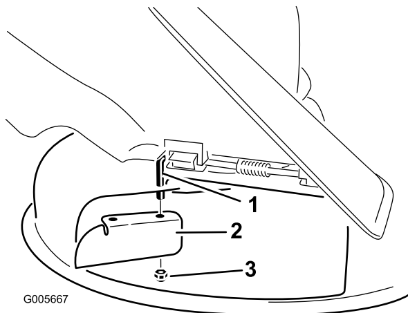
Bild 10 42 Zoll Mähwerk
