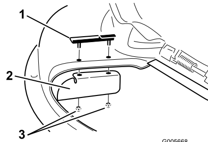
Bild 13 50 Zoll Mähwerk
