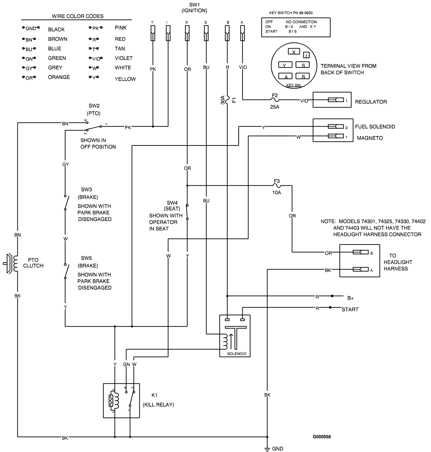
Schema elettrico (Rev. A)
