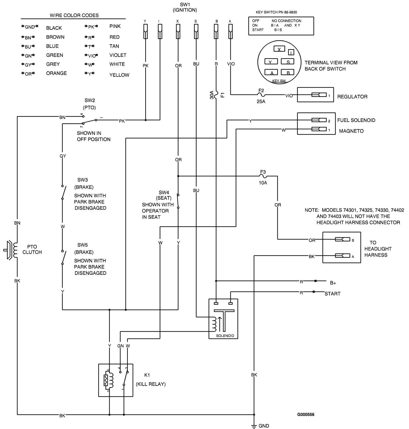
Elektrisches Schaltbild (Rev. A)
