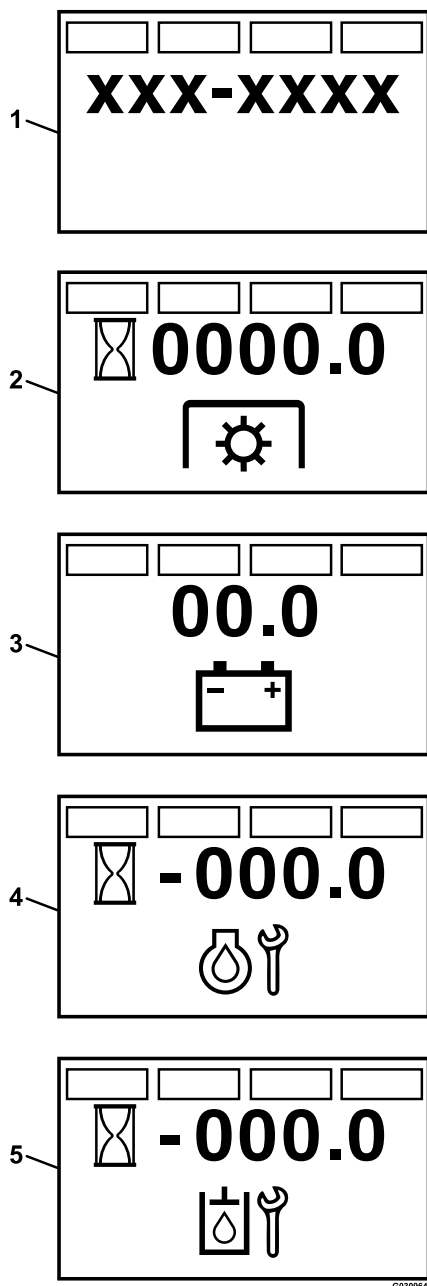
Figure 3 Écran d'accueil
