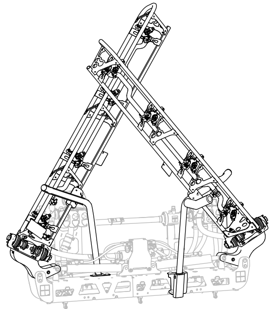
Figure 26 Position de transport en croix
