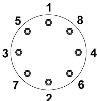
図 18 前輪
