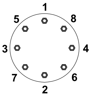
Рисунок 18 Передние колеса
