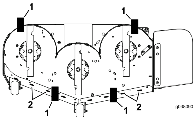
Figure 84 Vue inférieure
