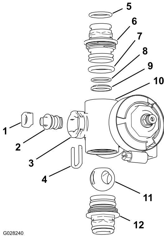
그림 130 섹션 밸브 매니폴드
