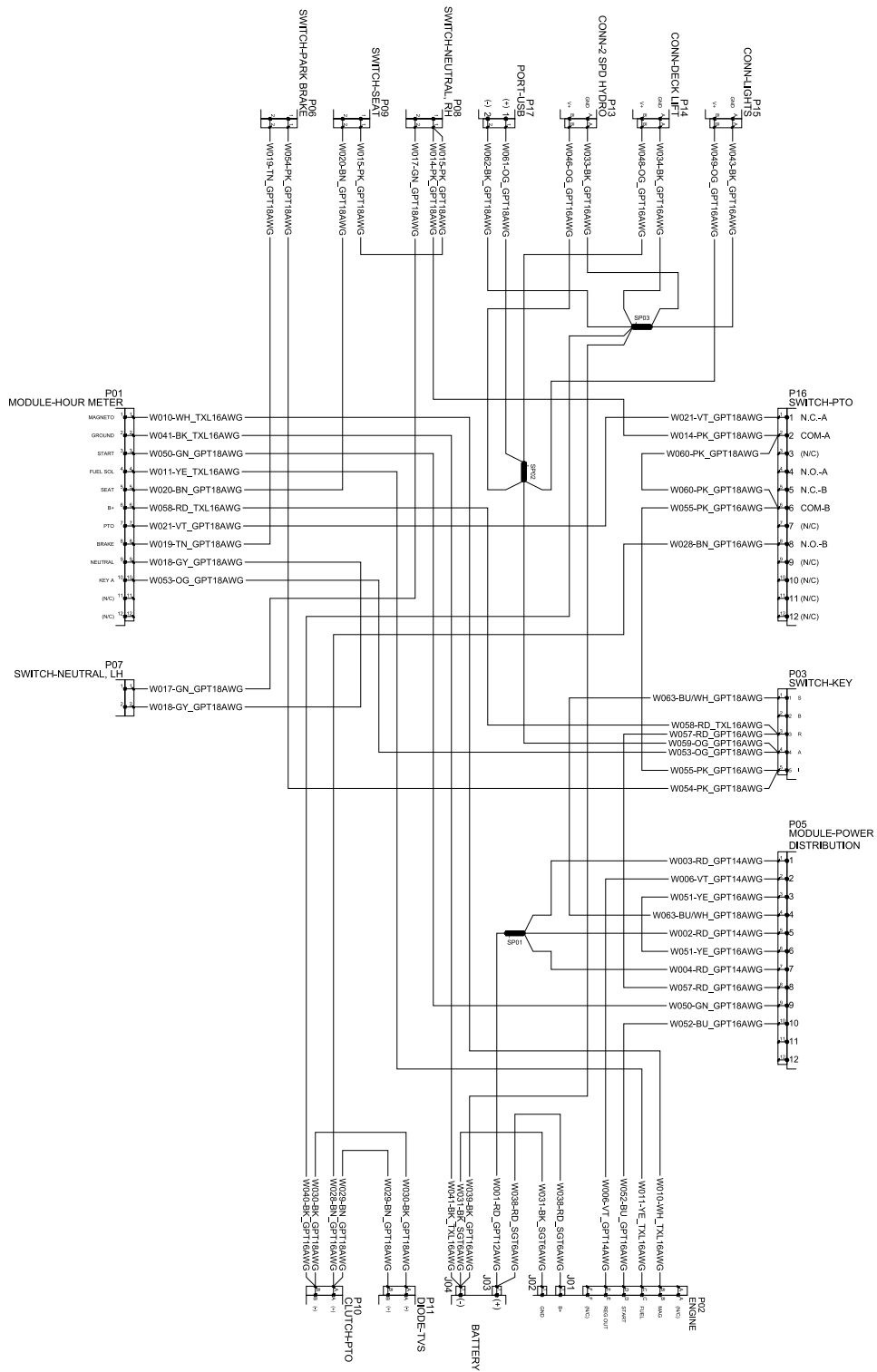
Elektronikkjema – side 2 (Rev. A)
