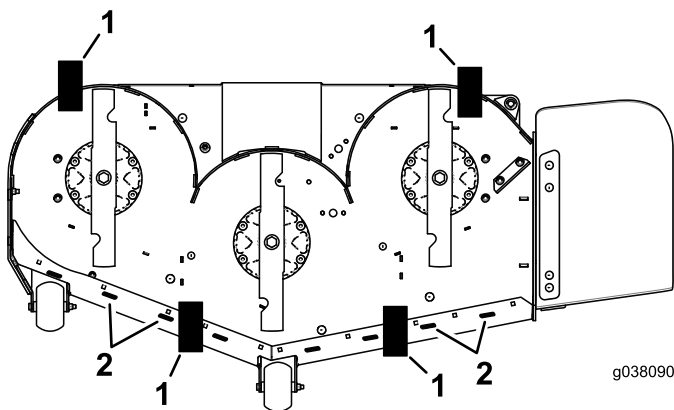
Figuur 83 Onderaanzicht
