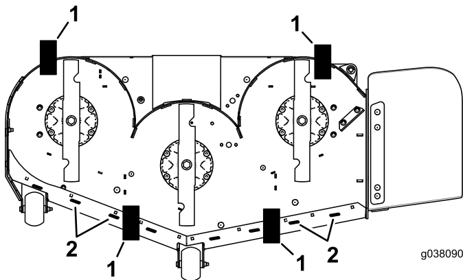
Figuur 83 Onderaanzicht
