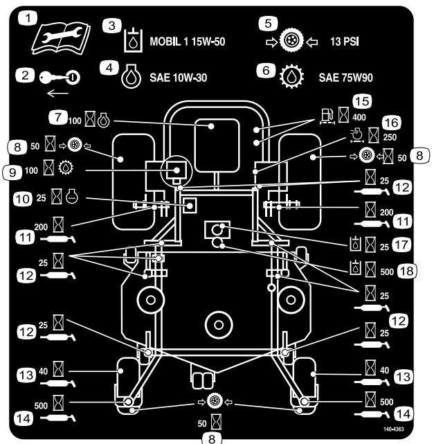
Figure 48 Modèles à éjection arrière
