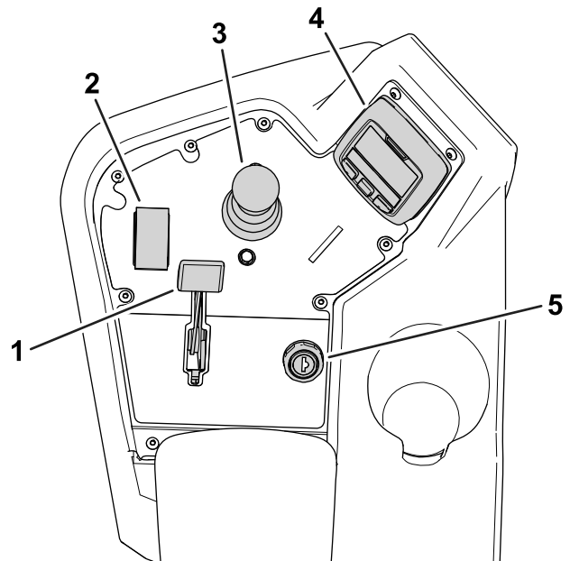
Figuur 14 Bedieningspaneel
