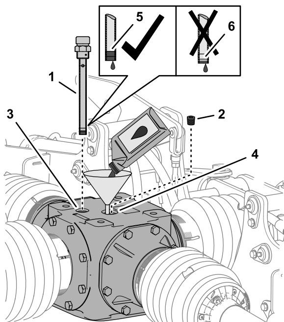
Рисунок 61 Средний редуктор
